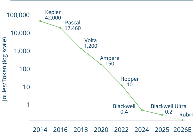
GPT-MoE-1.8T
